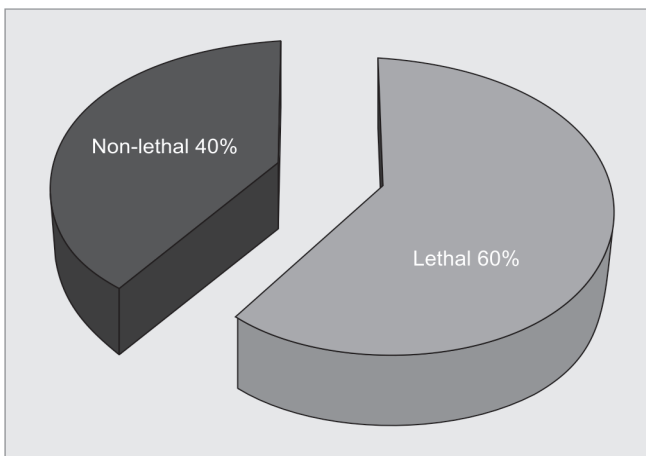
Fig. 6: Lethal/non-lethal anomalies
